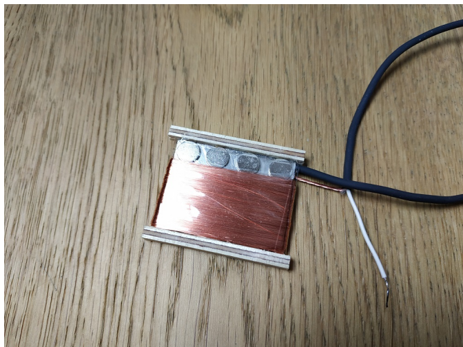
Alpen 4-String Single Coil mit hochpermeablem Nickel Kern
