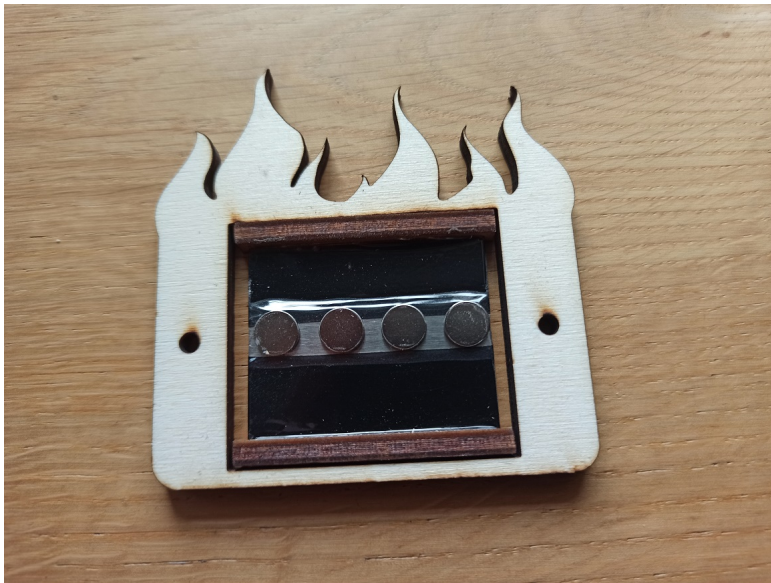
Montagerahmen Alpen Pickup Flame
