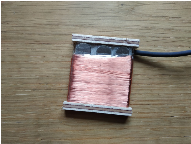
Alpen 3-String Humbucker mit hochpermeablem Nickel Kern
